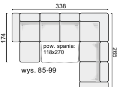
narożnik NAR.1OT/3W/H/2BF
