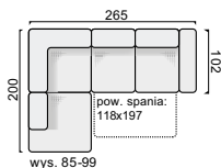
narożnik NAR.2OT/3W
