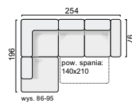
narożnik NAR.2OT/2R
