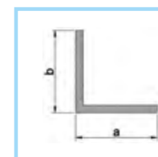
Prizma 022 L – профиль 20x40x1,2 мм
